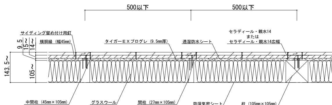
【サイディング縦張り（横胴縁）仕様】
