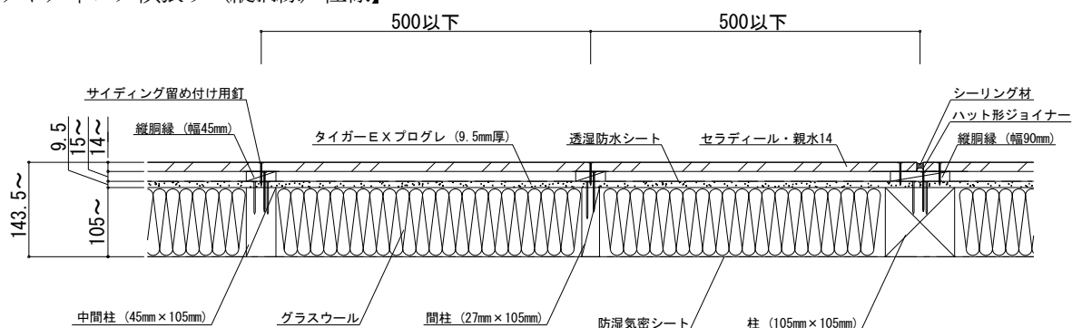
【サイディング横張り（縦胴縁）仕様】
